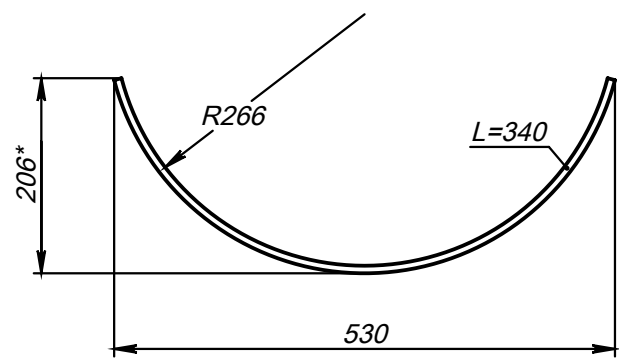
Поз.3 (Ложемент)
