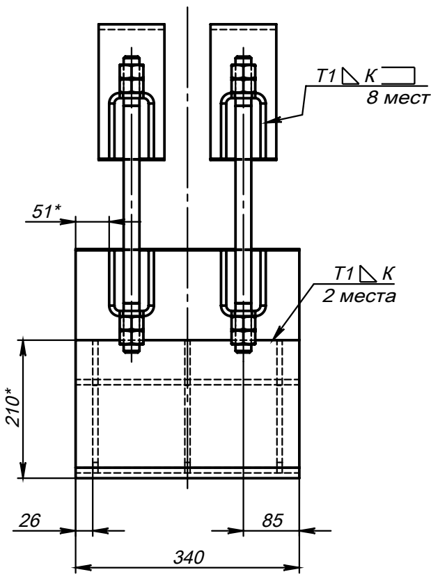
Поз.6 (Полухомут)
