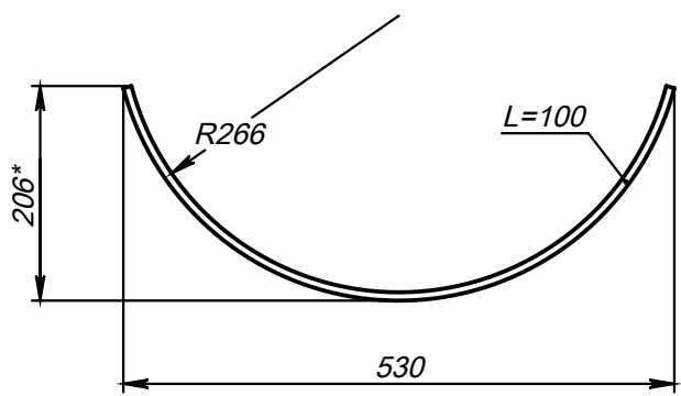
Поз.6 (Полухомут)
