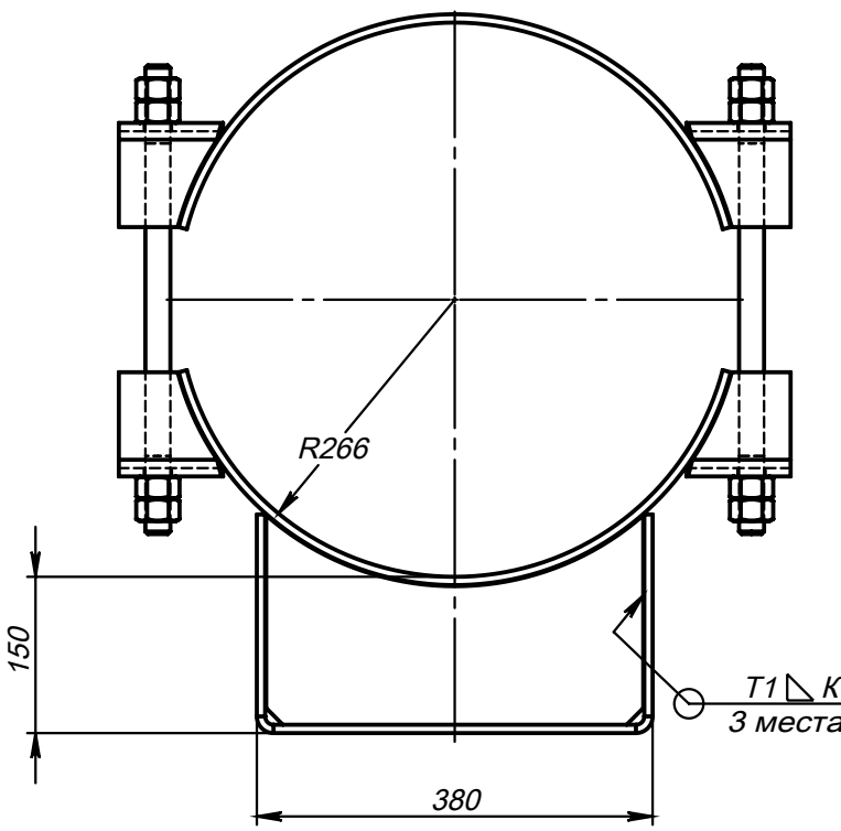
Поз.3 (Ложемент)
