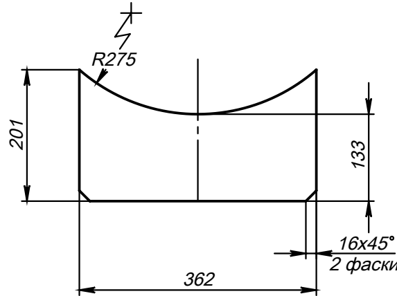
Поз.2 (Ребро)
